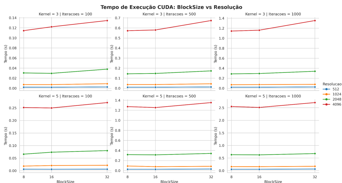
Figura 3 - Gráfico de Tempo de Execução CUDA: BlockSize vs Resolução
